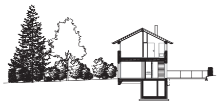
Schnitt
